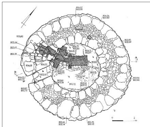
המבנה העגול – תכנית. מתוך : Kogan-Zehavi E. Atiqot 35: 135-142
